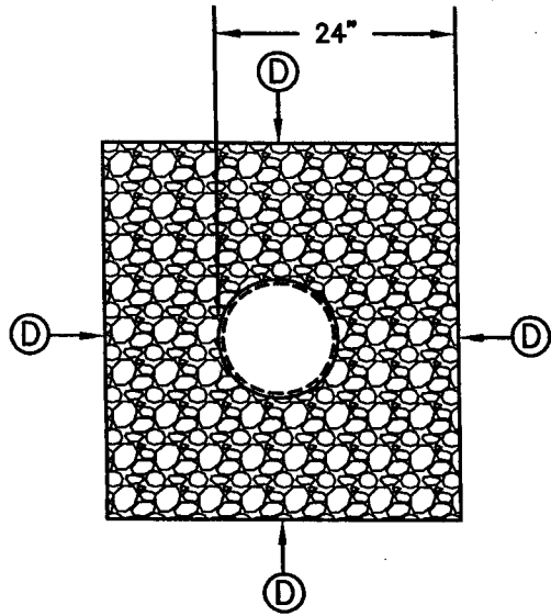
SECTION N.T.S.
